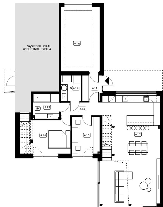
POZIOM 0
