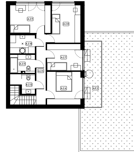
POZIOM 2
