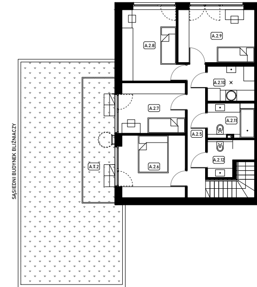
POZIOM 2
